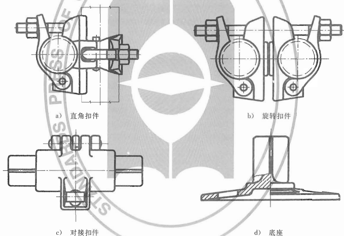
图 1 扣件型式示意图
