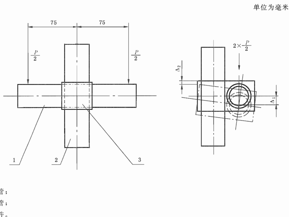
图 2 扣件抗滑性能试验示意图
